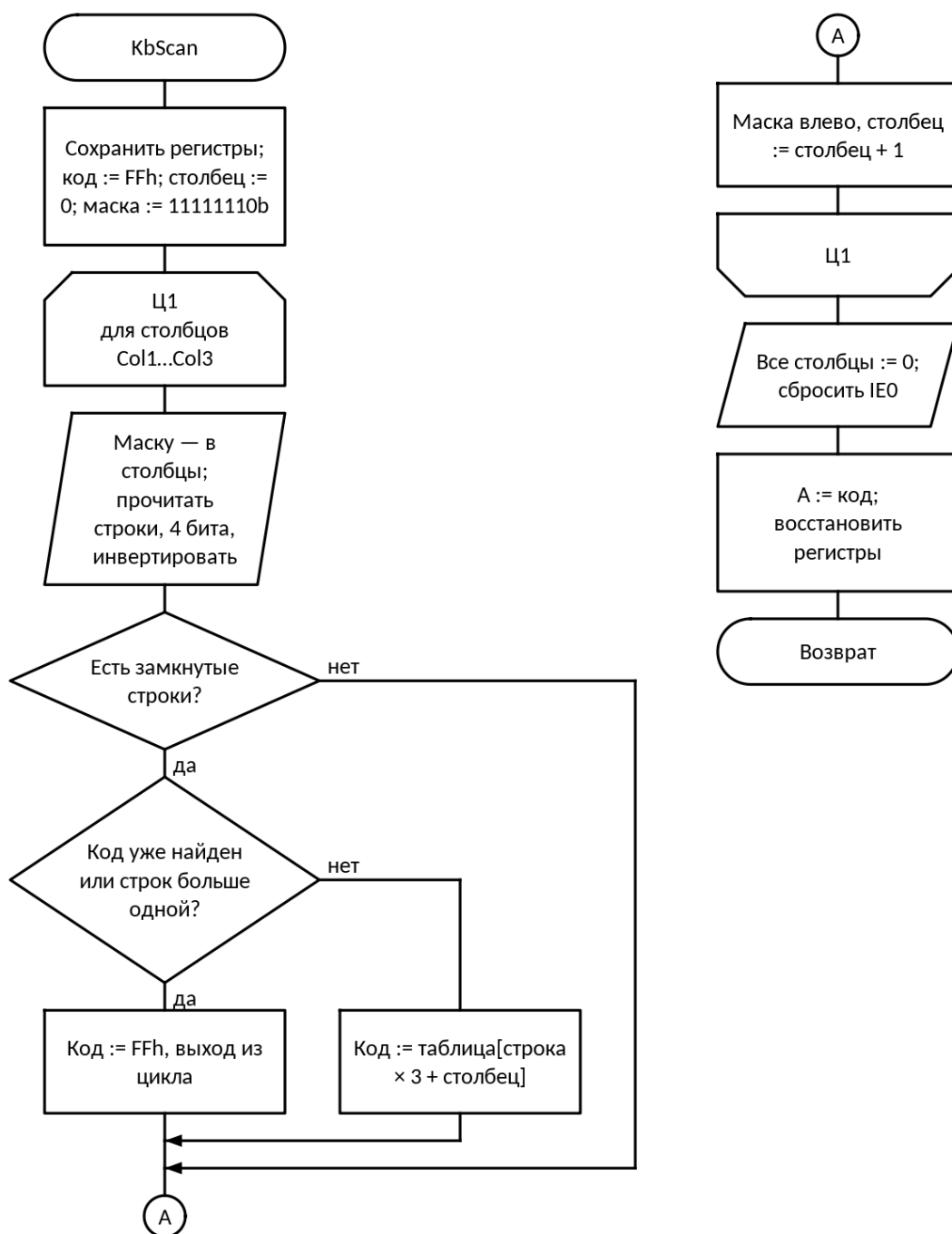
Рис. 3. Схема алгоритма: Опрос клавиатуры KbScan (обработчик INT0)
