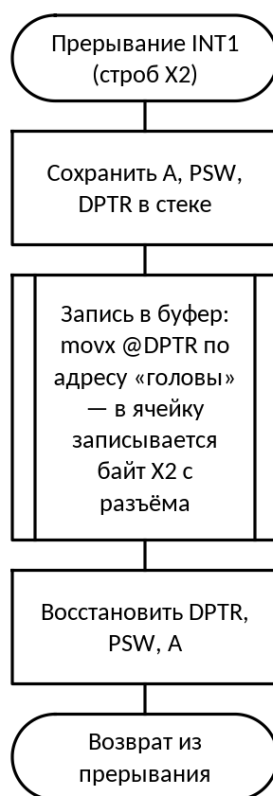
Рис. 6. Схема алгоритма: Обработчик прерывания INT1: приём отсчёта X2 от внешнего устройства
