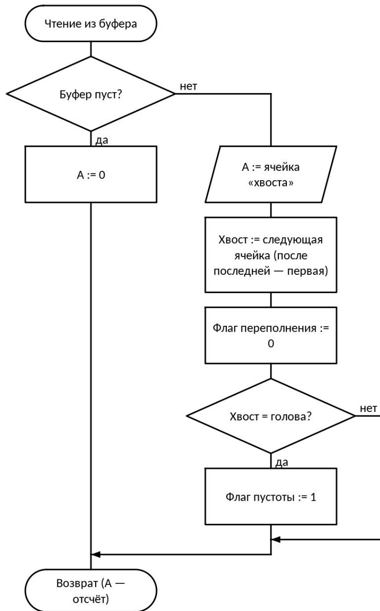
Рис. 7. Схема алгоритма: Чтение отсчёта из кольцевого буфера
