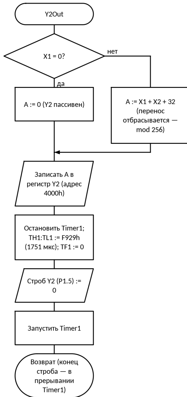
Рис. 12. Схема алгоритма: Расчёт и выдача сигнала Y2 (Y2Out)
