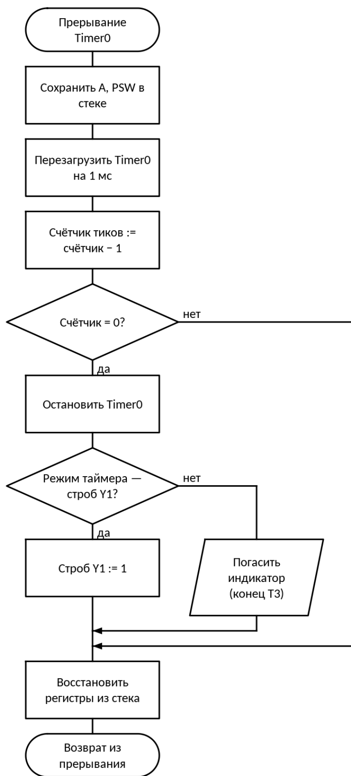
Рис. 10. Схема алгоритма: Обработчик прерывания Timer0: отсчёт T1 и T3
