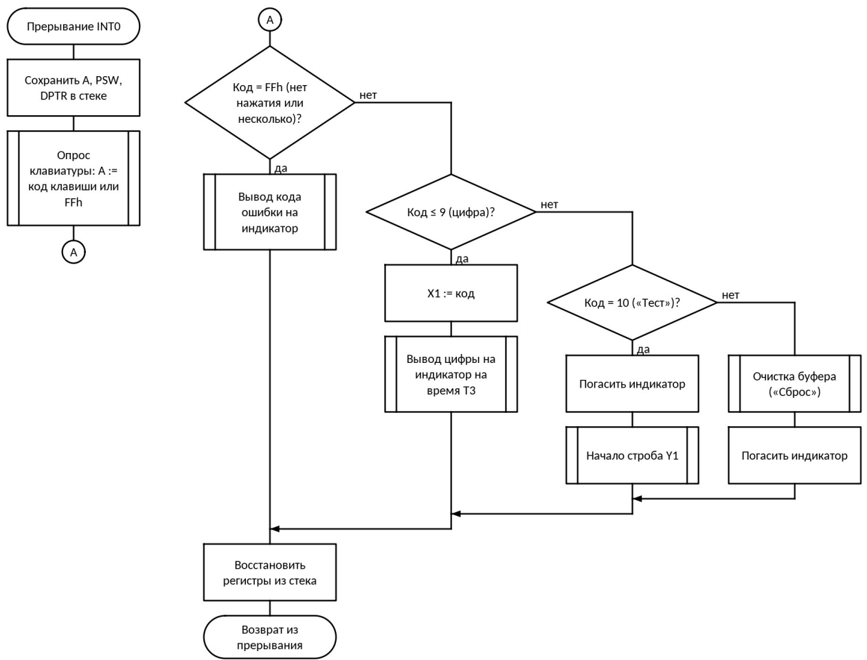
Рис. 4. Схема алгоритма: Обработчик прерывания INT0: реакция на клавишу
