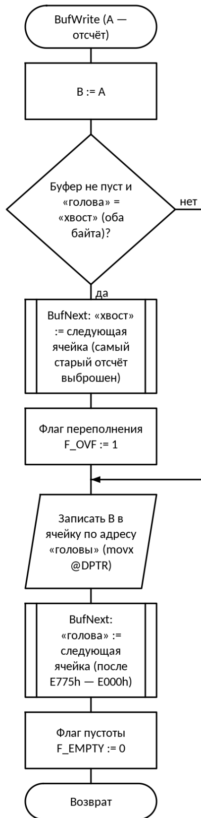
Рис. 5. Схема алгоритма: Запись отсчёта в кольцевой буфер BufWrite
