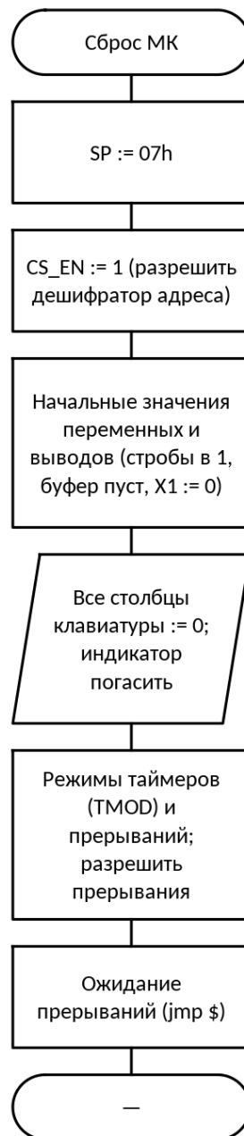
Рис. 1. Схема алгоритма: Инициализация МПС и основная программа
