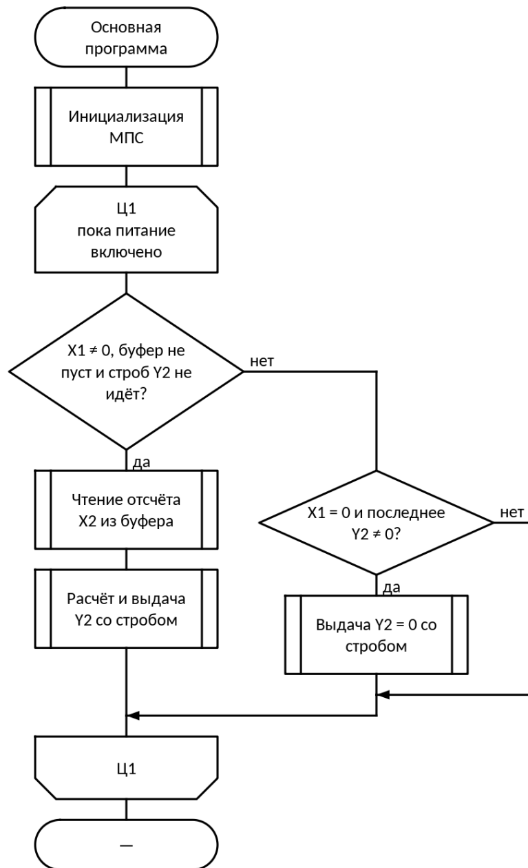
Рис. 2. Схема алгоритма: Основной цикл программы
